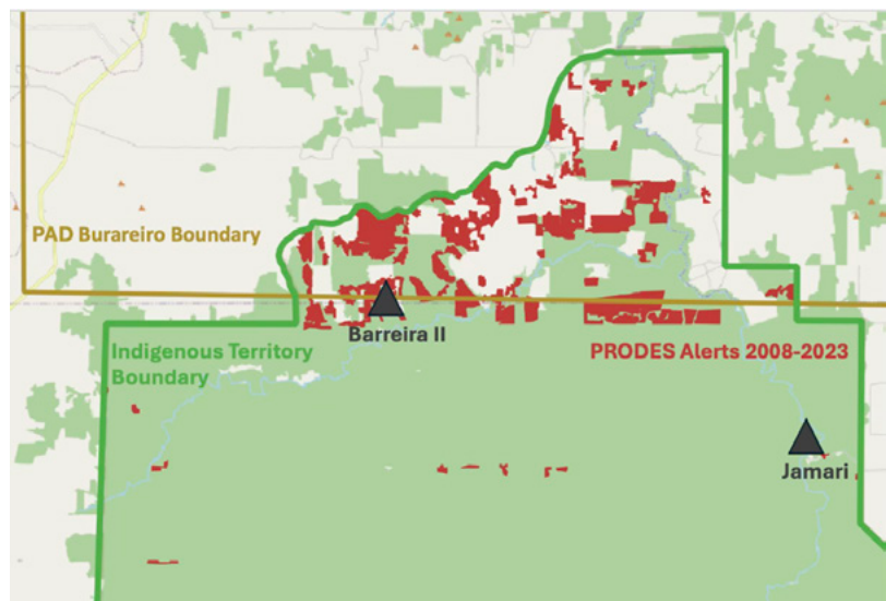
Desmatamento de 2008 a 2023 na área do PAD Burareiro, dentro do território Uru-Eu-Wau-Wau em Rondônia, Brasil. PRODES, 2025
